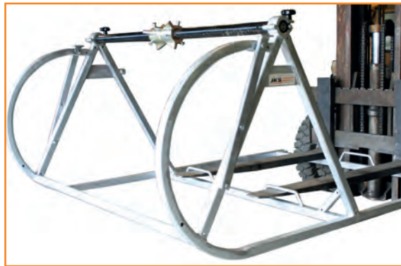
Tyhjän pukin liikuttelu onnistuu vaivattomasti vaikkapa trukilla
