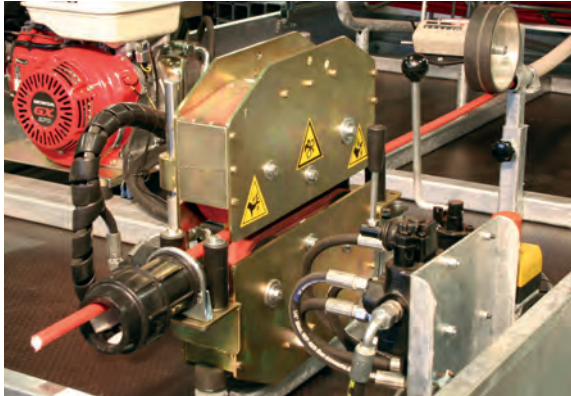
Hydraulisella puristuksella varustettu PPD 402 -välivetolaite putkikäärmevaunussa.
