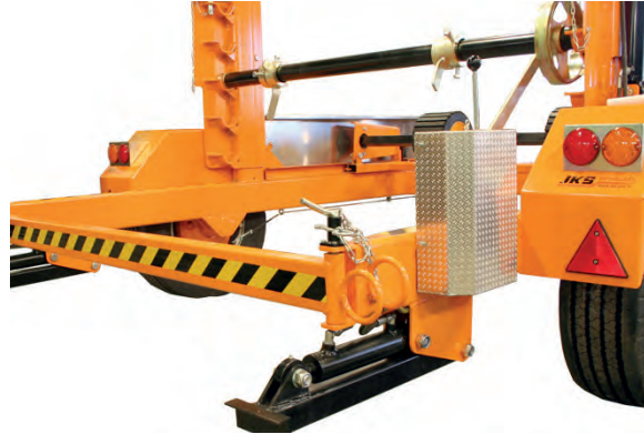
Portaattomasti säätävät takatukijalat on helppo säätää maaston mukaan.
