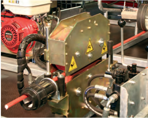
Hydraulisella puristuksella varustettu PPD 402 -välivetolaite takaa nopean ja sujuvan vedon.
