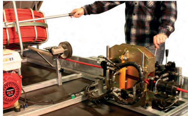
Kelan käsijarru ja muut keskeiset hallintalaitteet suoraan käyttäjän ulottuvilla.
