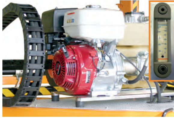
Hydraulikoneikko + 13hp Honda + öljylämpö-/määrämittari - määrä ja lämpö yhdellä vilkaisulla
